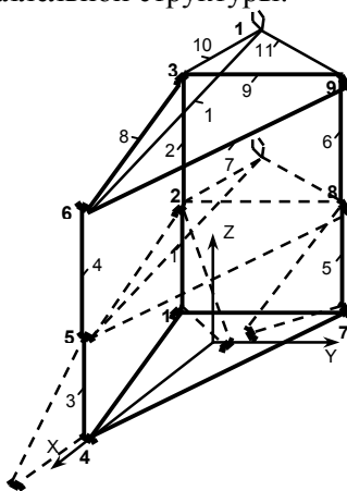
Рисунок 3 – Манипулятор параллельной структуры
